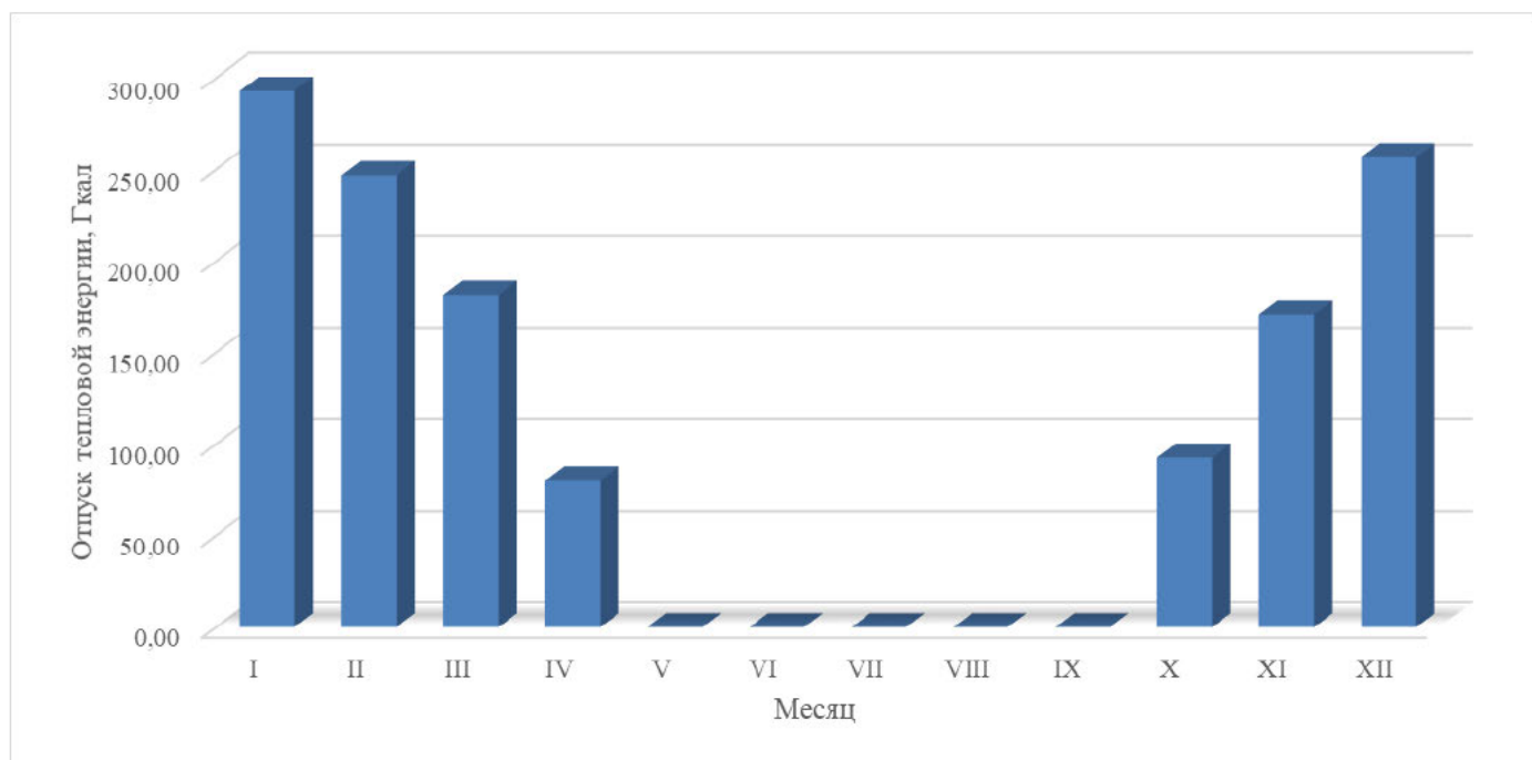
Рисунок 1.4 – Оптимальный температурный график отпуски тепловой энергии котельной «№2»
