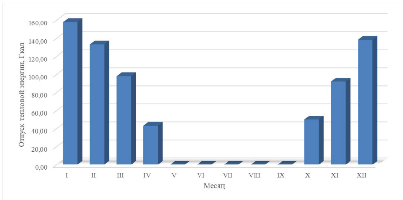
Рисунок 1.3 – Оптимальный температурный график отпуски тепловой энергии котельной «№1»
